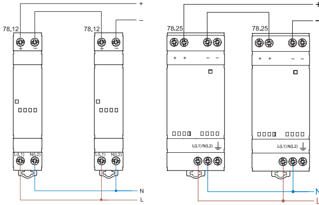
串聯連接
