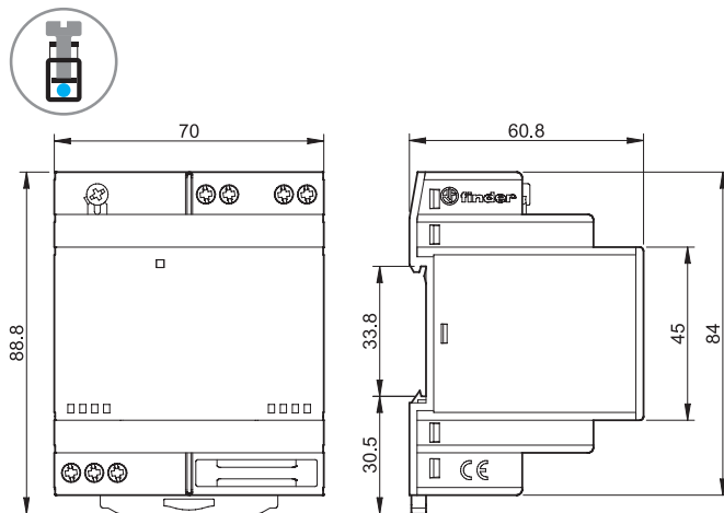
78. 51 / 78. 61 螺絲端子
